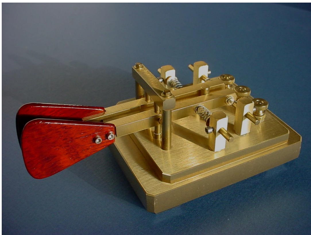
Pastička jambická WE4S
