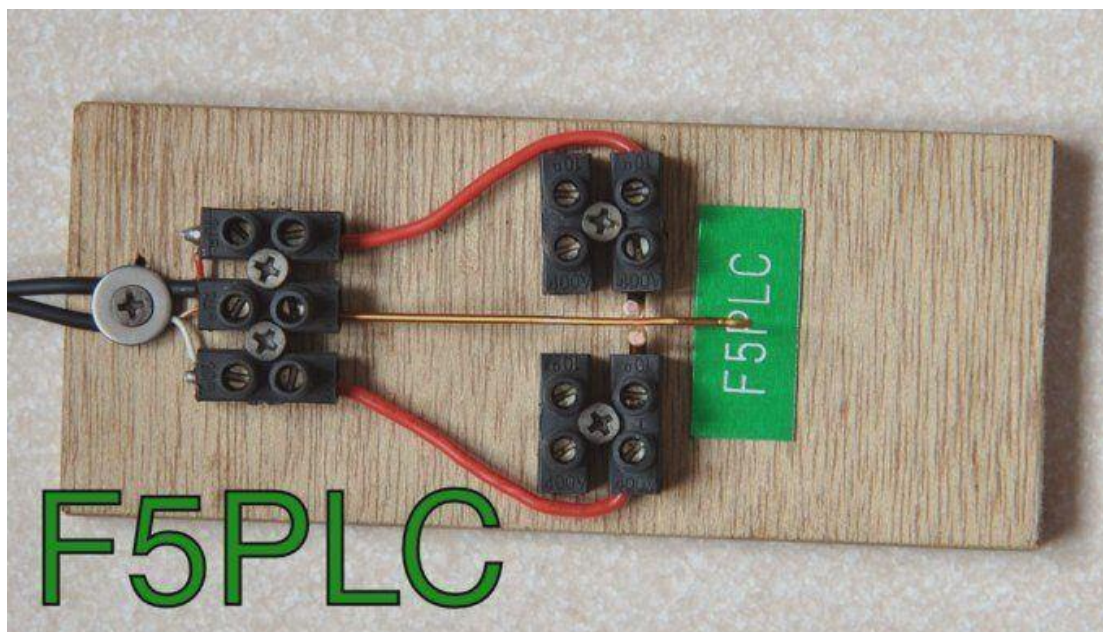
Pastička jednopáčková z elektrických svoriek podľa F5PLC
