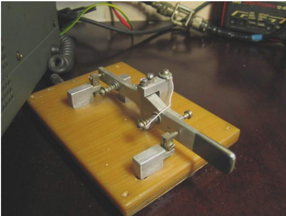
Pastička jednopáčková YL2RMK
