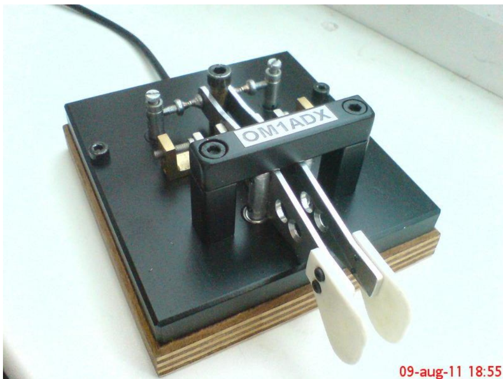
Pastička jambická magnetická OM1ADX http://www.radio-foto.eu/radio/klic.php
