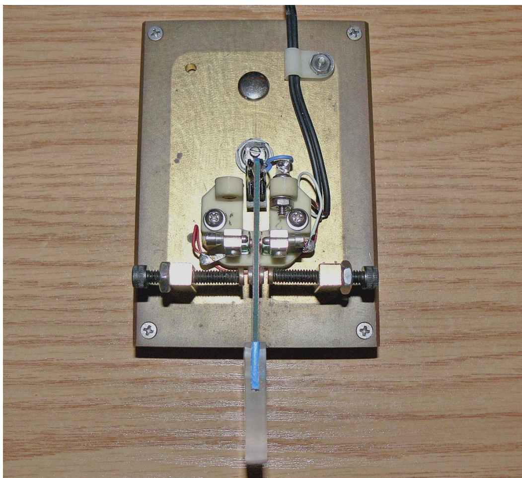
Pastička jednopáčková z plošného spoja a polarizovaného relé podľa N2HO
