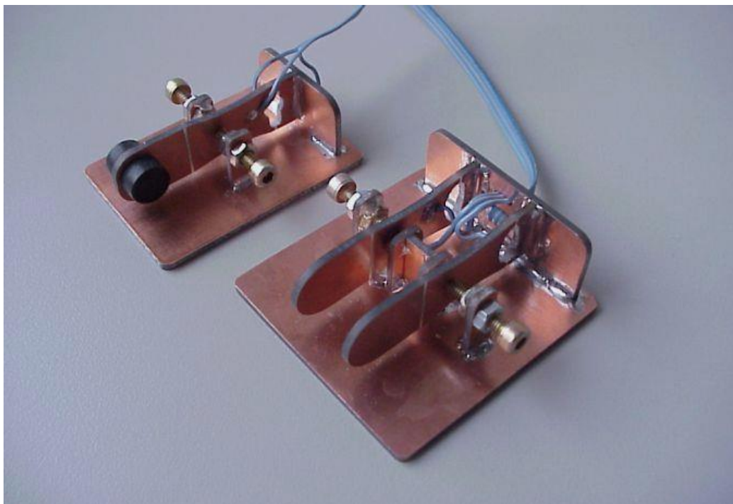
Pastičky jednopáčková a jambická z plošného spoja podľa PA0CMU http://members.ziggo.nl/cmulder/paddle.htm
