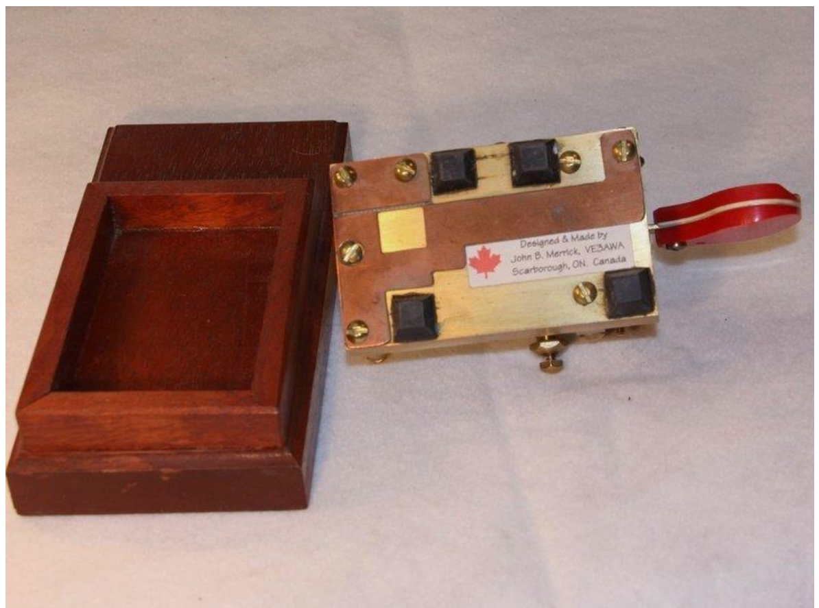
Pastička jednopáčková VE3AWA, s dreveným podstavcom
