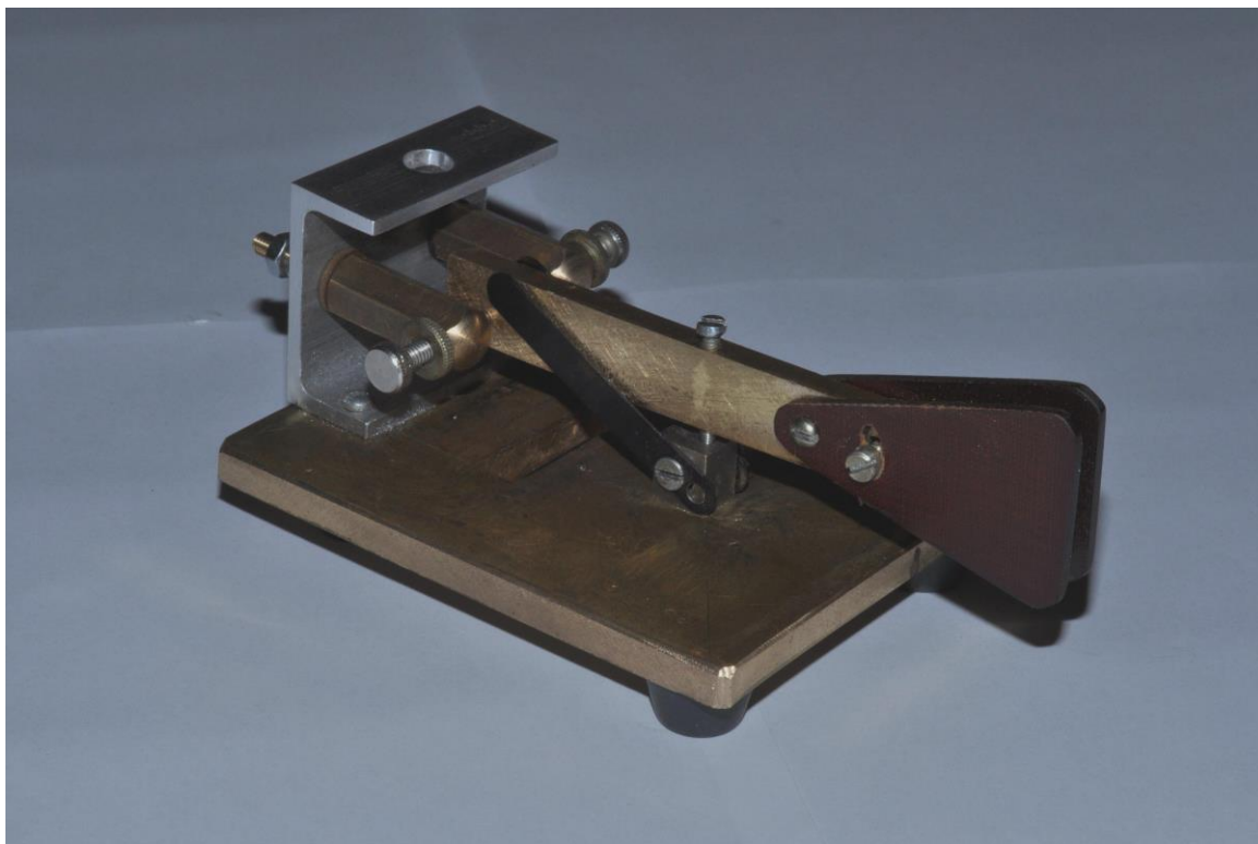
Pastička jednopáčková, robustná, má dve ploché perá, navrhnutá Valerijom, UA3AO
