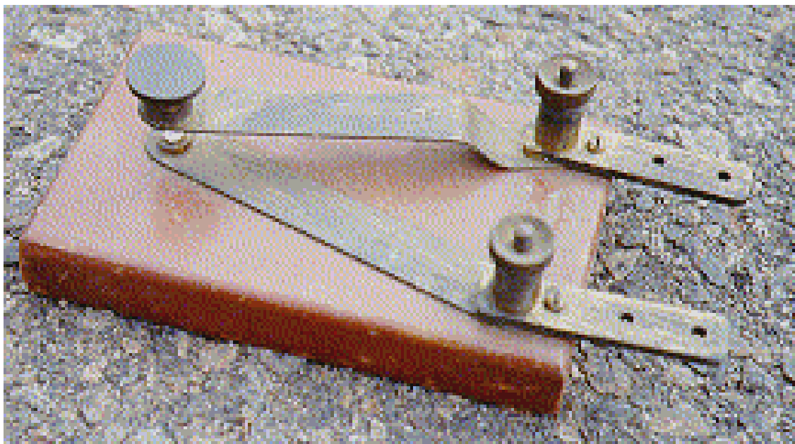
Jednoduchý ručný kľúč z plochého pera
