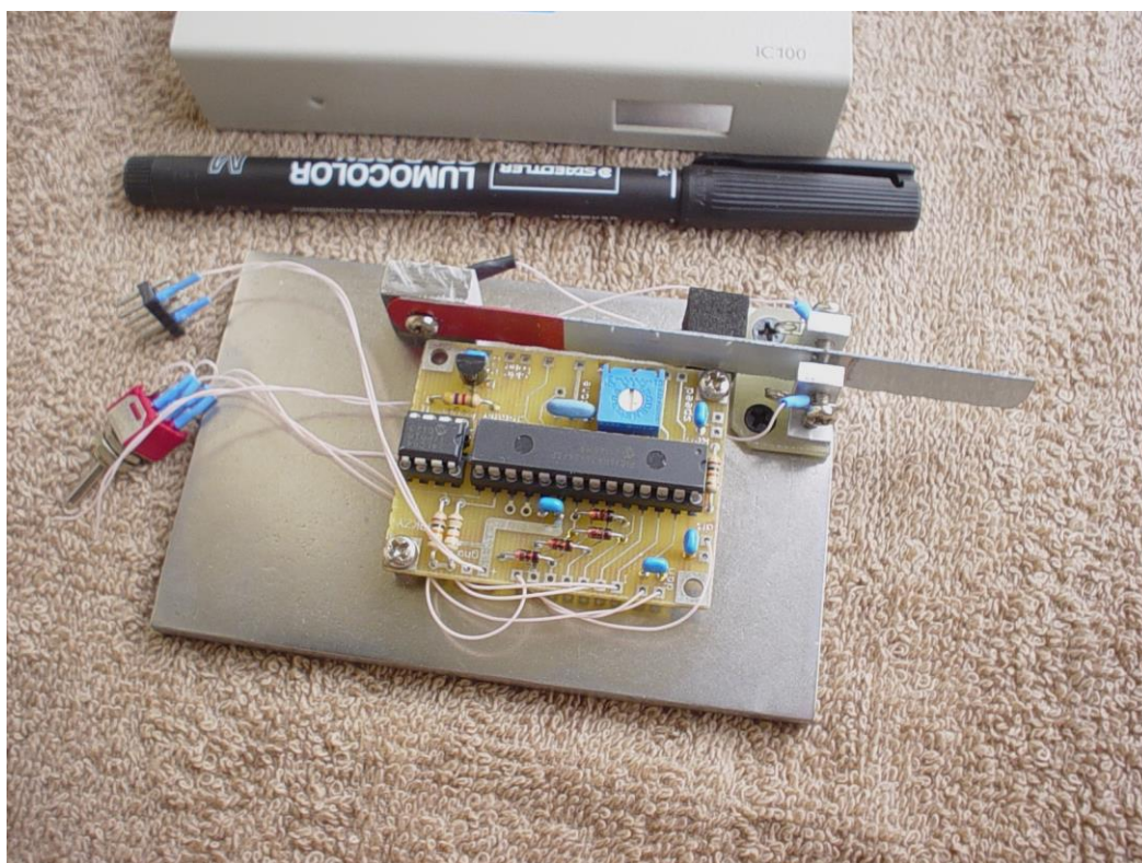
Pastička jednopáčková z plochého pera, elbug podľa VE3IVM
