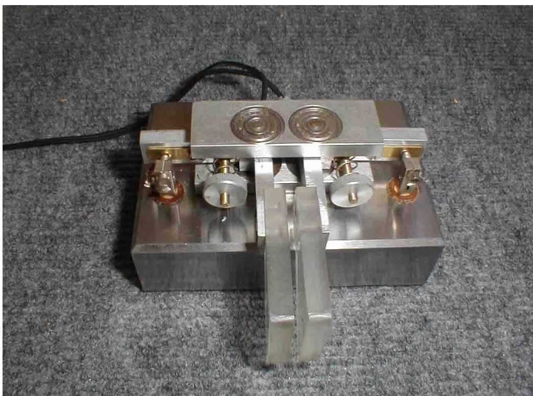
Pastička jambická OM3WAT, slovenský KENT
