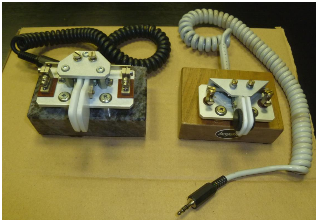
Pastičky jambické OM3TC
