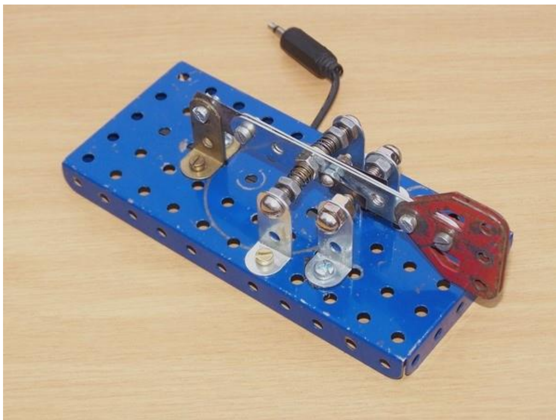
Pastička jednopáčková cootie key G4ZXXN
