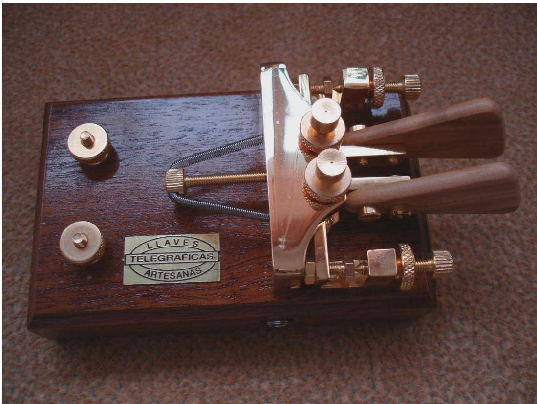
Pastička jambická EA6YG
