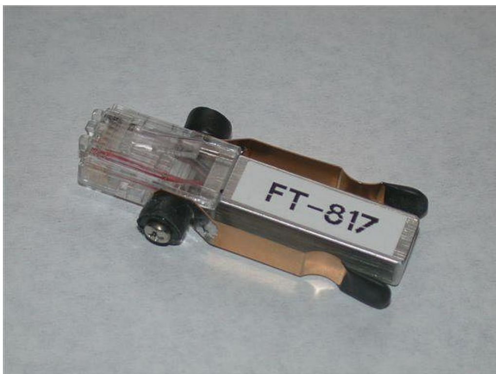
Pastička jambická miniatúrna s konektorom pre YAESU FT-817
