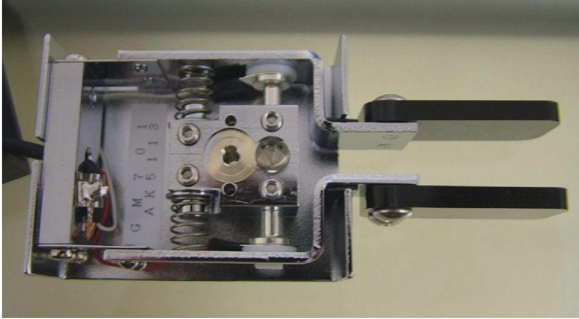
Pastička jambická prenosná GHD
